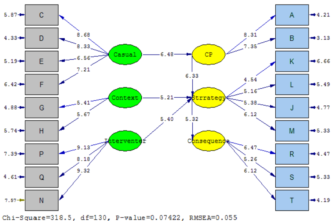
شکل ۲. مدل نهایی پژوهش به همراه ضرایب استاندارد
